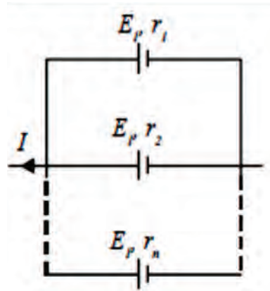
Sumber: Dokumen Kemdikbud Gambar 5.31 Rangkaian Elemen Secara Paralel
