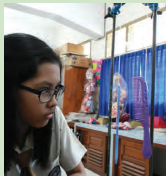
Gambar 5.1 Dua Sisir Bermuatan yang digantung
