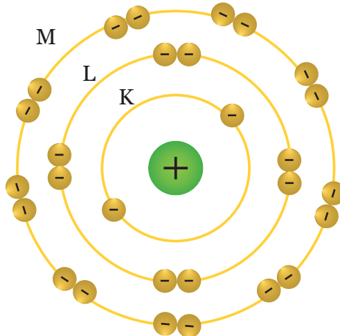
Gambar 4.15 Tingkat Energi Atom dan Jumlah Elektron Maksimal
