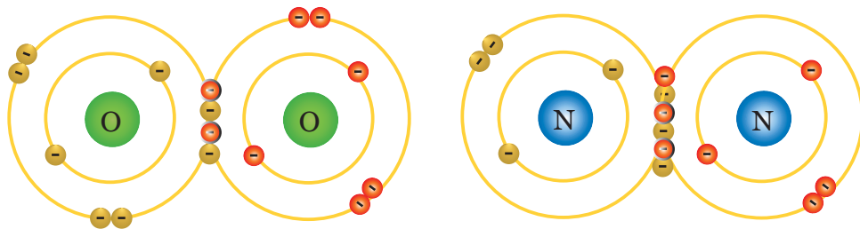
Sumber: Dokumen Kemdikbud Gambar 4.21 Penggunaan Bersama Elektron pada (a) Gas Oksigen (O 2 ) dan (b) Gas Nitrogen (N 2 )
