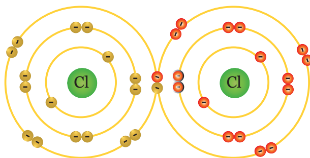
Sumber: Dokumen Kemdikbud Gambar 4.20 Penggunaan Bersama Dua Elektron pada Molekul Cl 2
