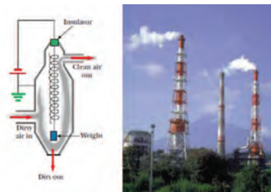
Gambar 5.44 Cerobong Asap
